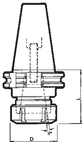
DIN 69871-AD + B
