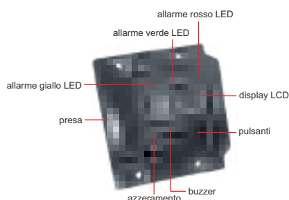
IST-04TT350 tipo A
