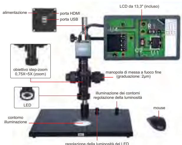
ISM-DL301 (con illuminazione dei contorni)
