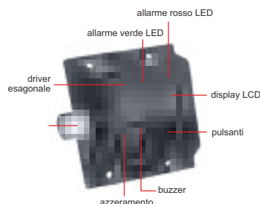
IST-04TT815 tipo B
